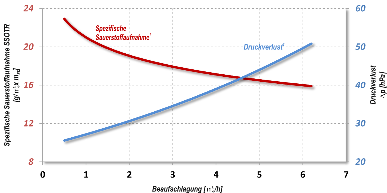
Spezifischer Sauerstoffeintrag und Druckverlust OXYFLEX® - MT235
