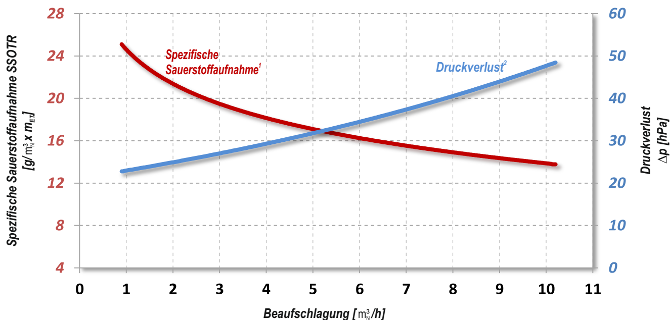
Spezifischer Sauerstoffeintrag und Druckverlust OXYFLEX® - MT300
